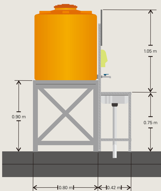
POTONGAN B
